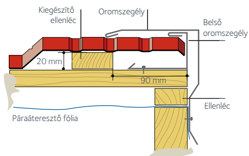
2 A tetőzet oldalának a részei
